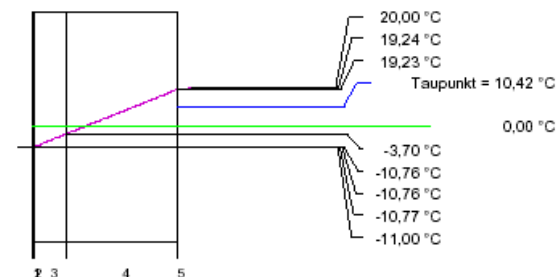
Dicken - Diagramm Temperaturverteilung
